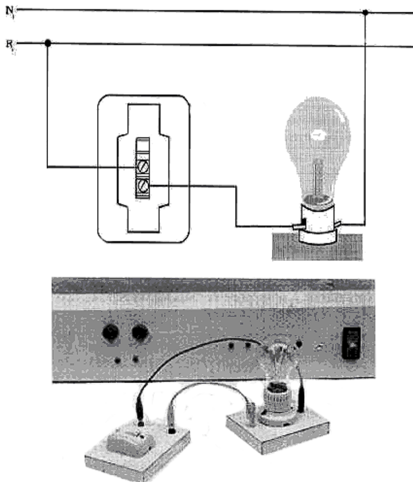
Figura 58: Diagrama funcional
