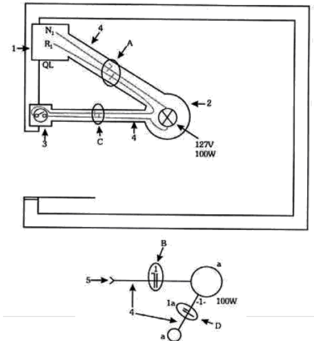
Figura 59: Esquema unifilar
