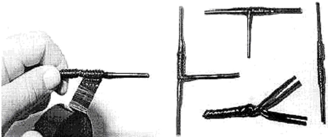
Figura 52: Completando com segunda camada da fita isolante
