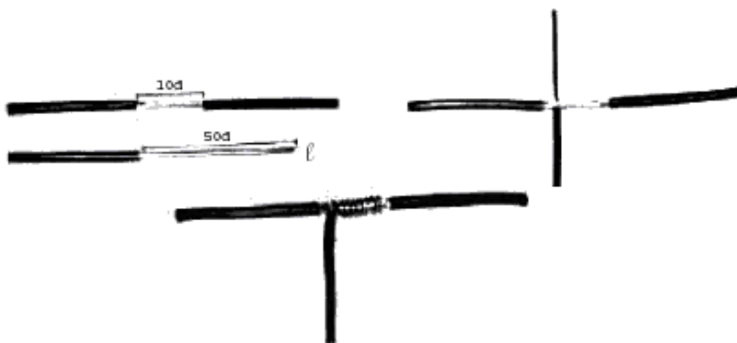
Figura 36: Emenda de um condutor flexível com um rígido
